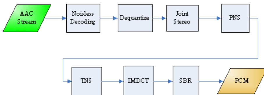
AAC解码流程图
