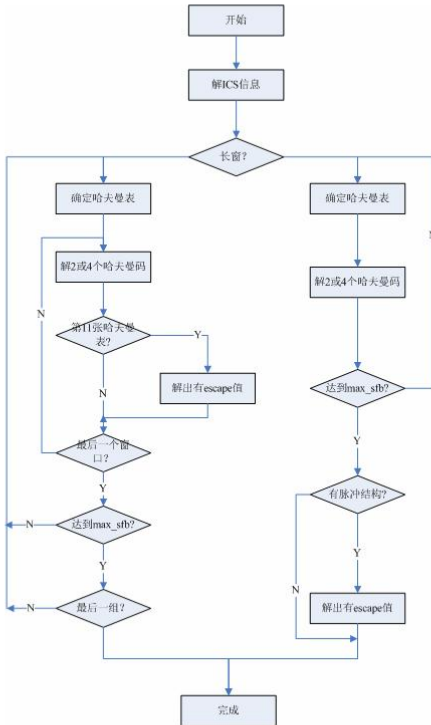
无噪声解码流程图
