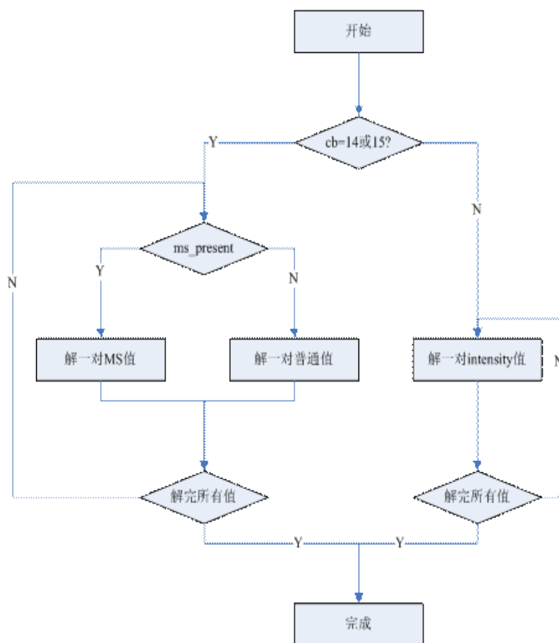
联合立体声解码流程图
